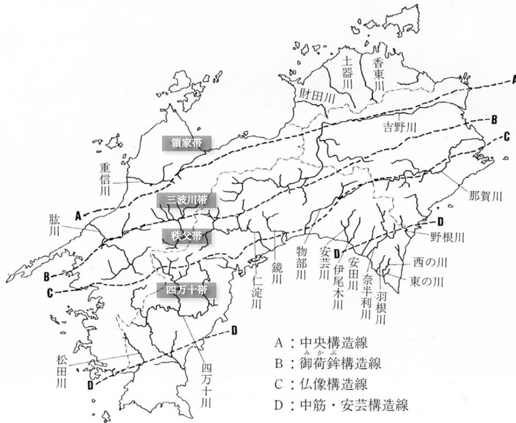
図 1-4 四国の地質構造線と河川
