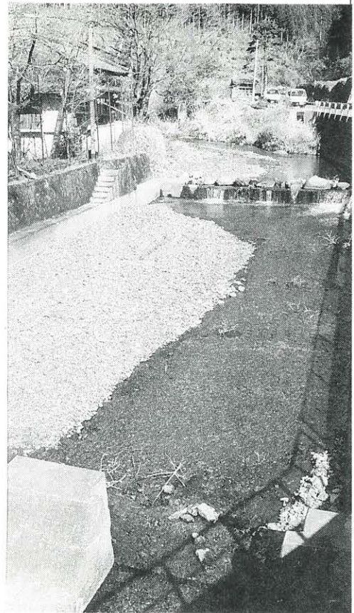
▲手前のコンクリートの間へ木の角材を渡して水をせき止め河川プールとした
