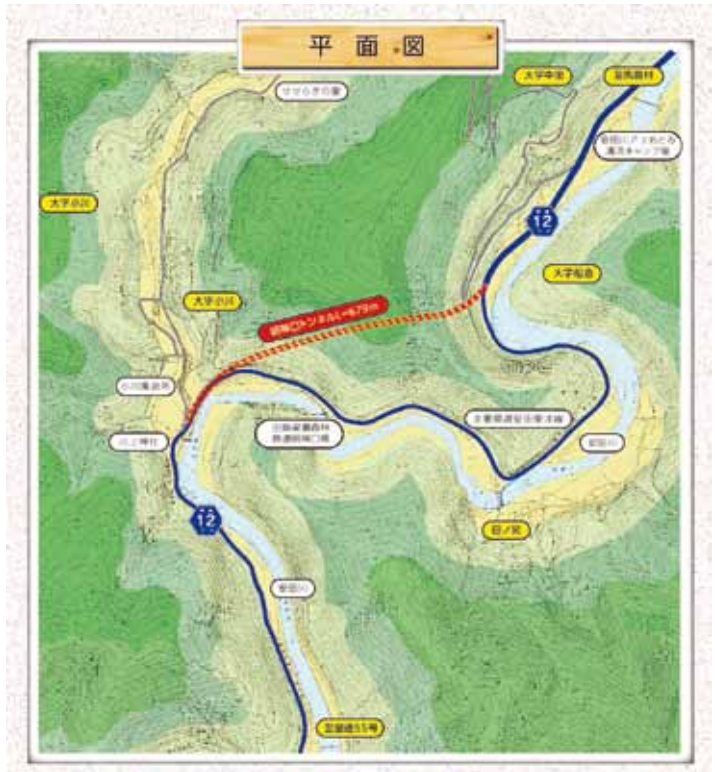
▲ 明神口トンネルの平面図
