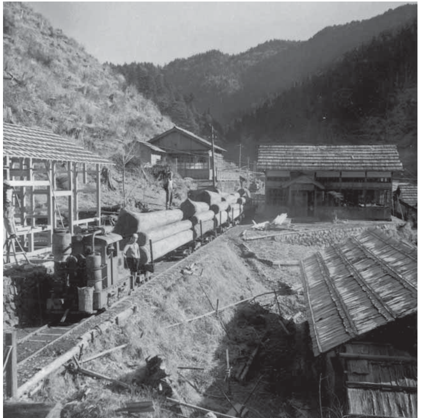
右 / 昭和 26 年の魚梁瀬署東川軌道搬出、と写真説明にある。東川事業所の一帯だろう。右奥が事務所、その左上が主任の宿舎、左手前建築中の建物は発電小屋と思われる。屋根は杉皮ぶきであろう。戦後まもなくで、機関車は木炭ガス車と見られる。前ステップには炭ラスらしきものが載っている。=寺田正写真文庫提供
